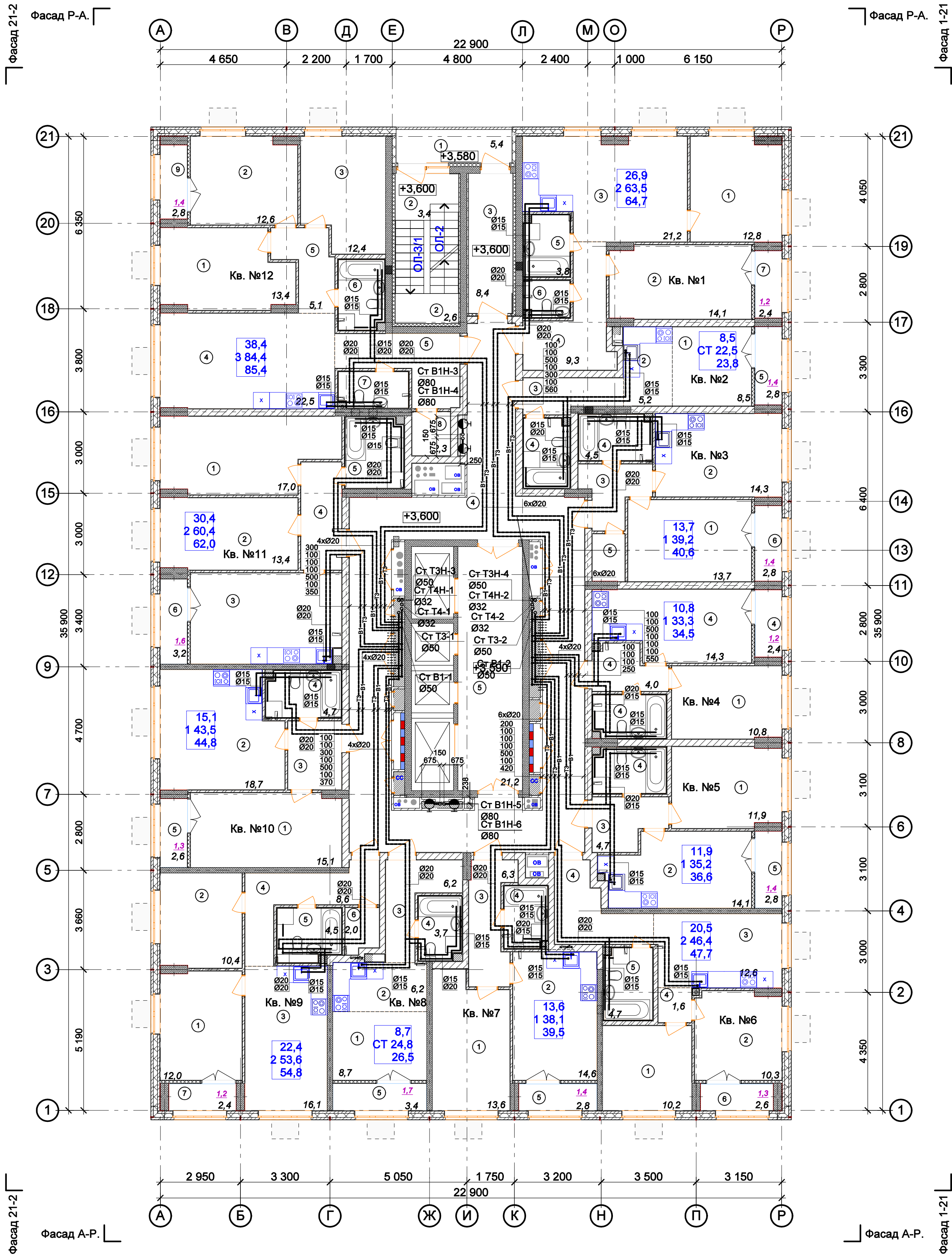
План 2 этажа с сетями водоснабжения
