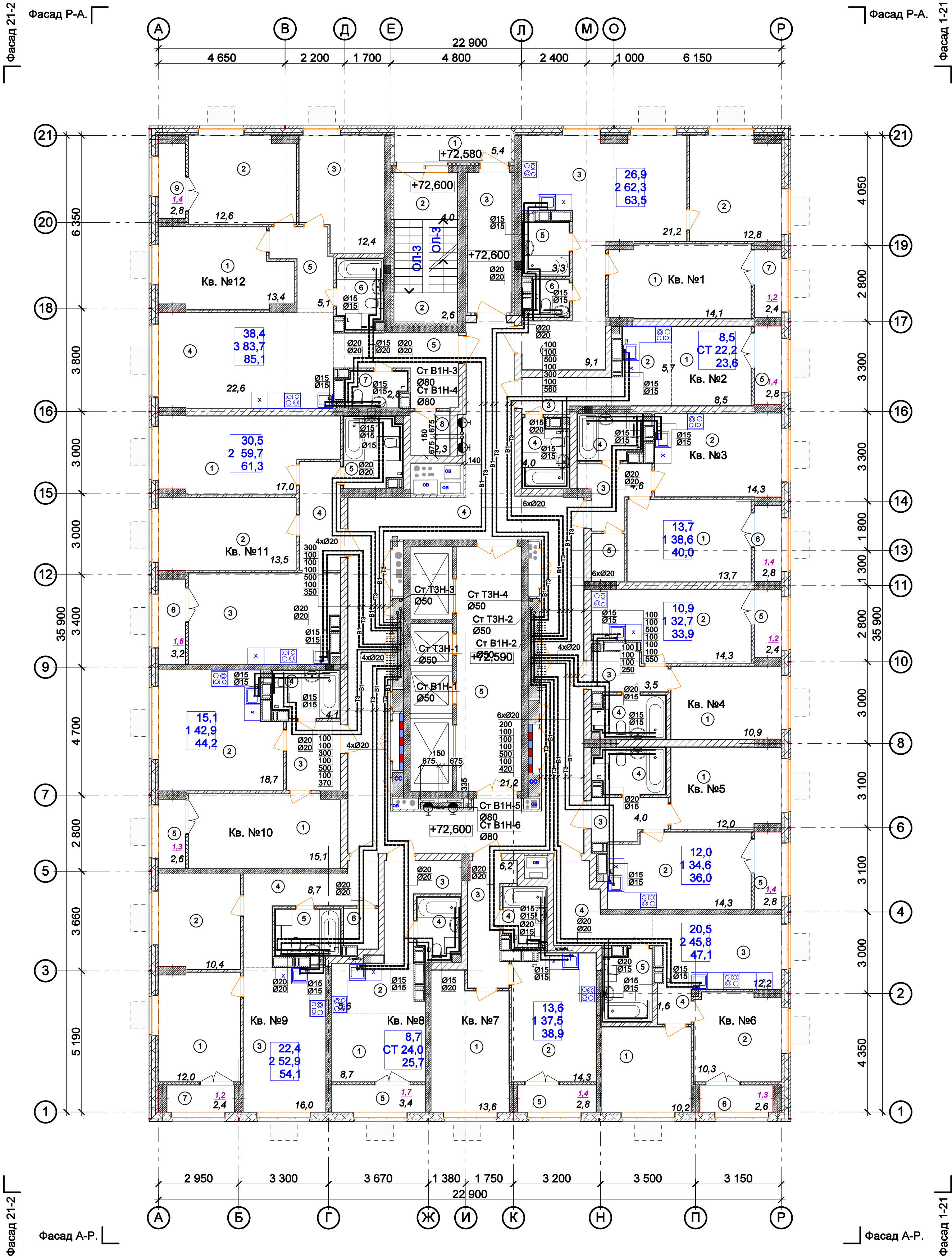
План 18-25 этажей с сетями водоснабжения
