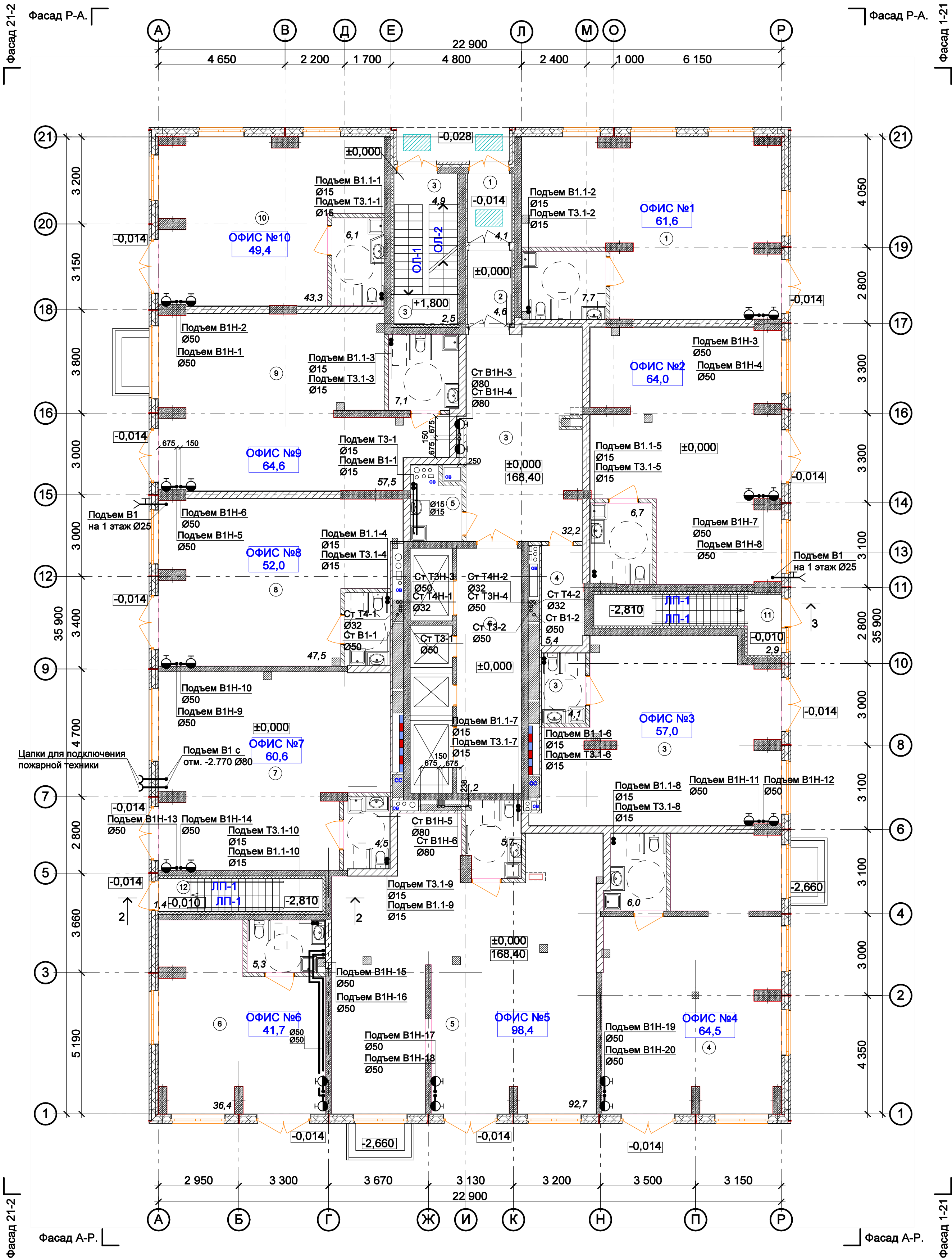
План 1 этажа с сетями водоснабжения
