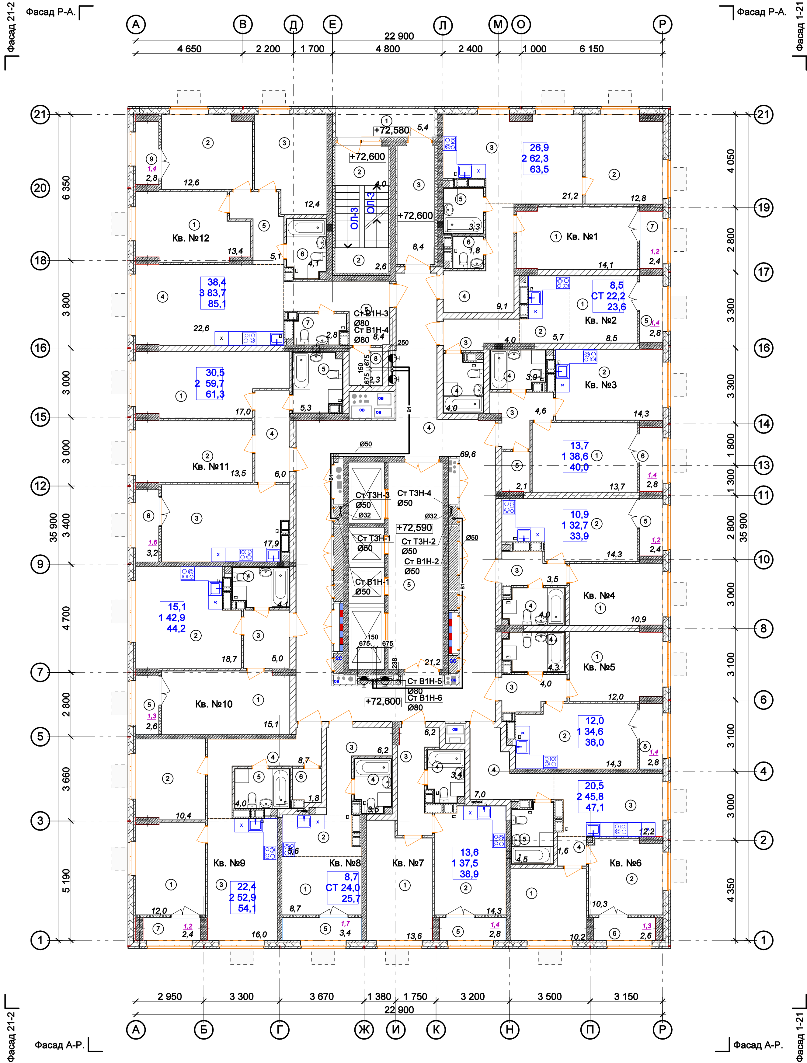
План 25 этажа с сетями водоснабжения (верх)
